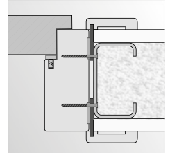
montáž na vruty do stěny ze sádrokartonu
