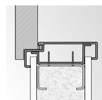
rohová zárubeň velká montáž na sádrokartonovou stěnu
