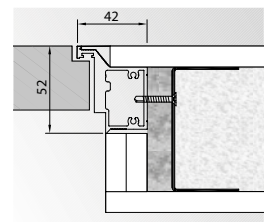
Bezpolodrážkové standard (otevírané ven)
