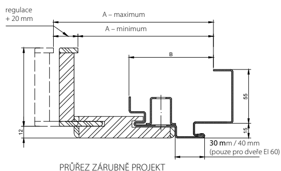
PRŮŘEZ ZÁRUBNĚ PROJEKT
