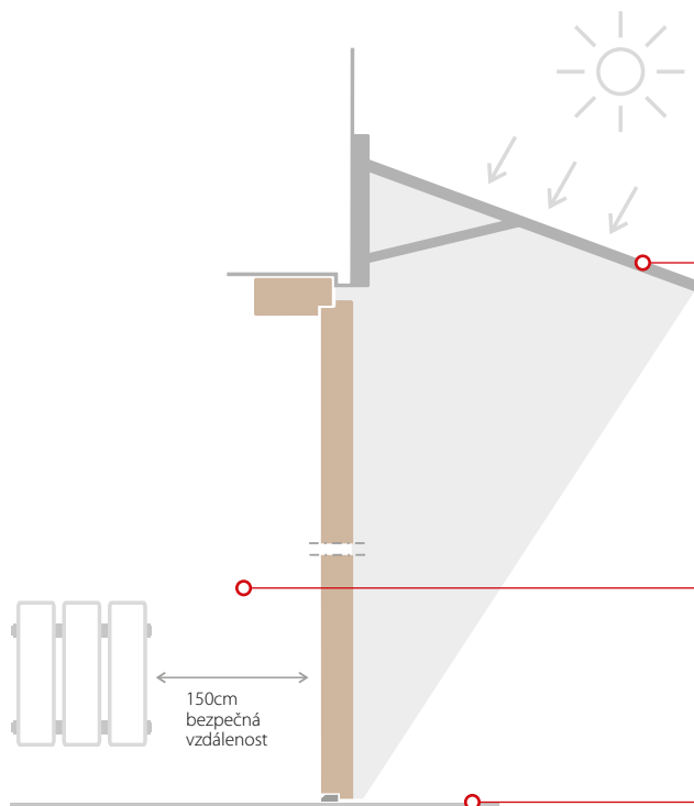
Názorný výkres
