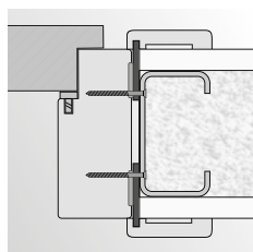
montáž na vrtvy do stěny ze sádrokartonové desky
