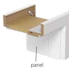
Porta SYSTEM + Regulující panel*
